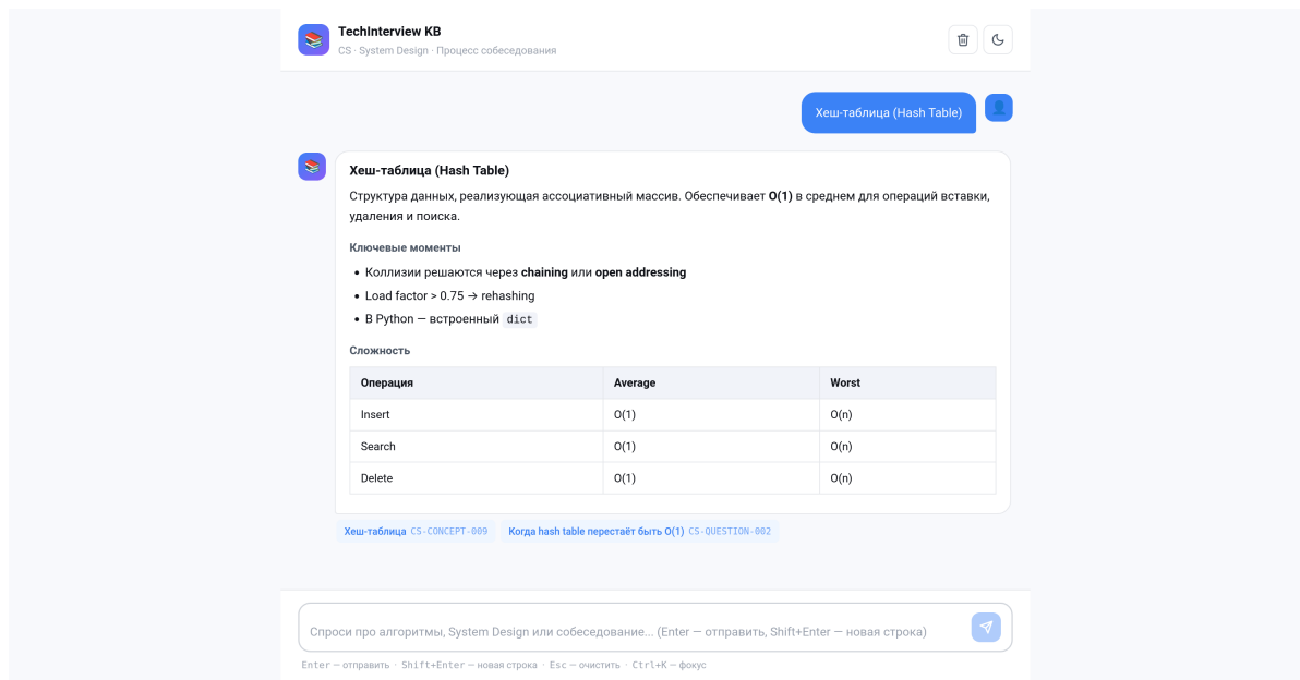
Рисунок 3.4 – Взаимодействие с MVP: выбор предложенного вопроса, рендеринг Markdown-ответа и отображение метрики уверенности
