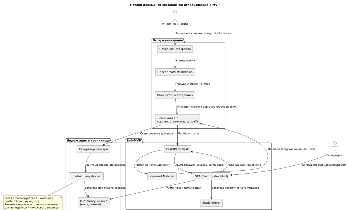
Рисунок 3.3 – Диаграмма потоков данных: от создания единицы знаний до использования в веб-MVP
