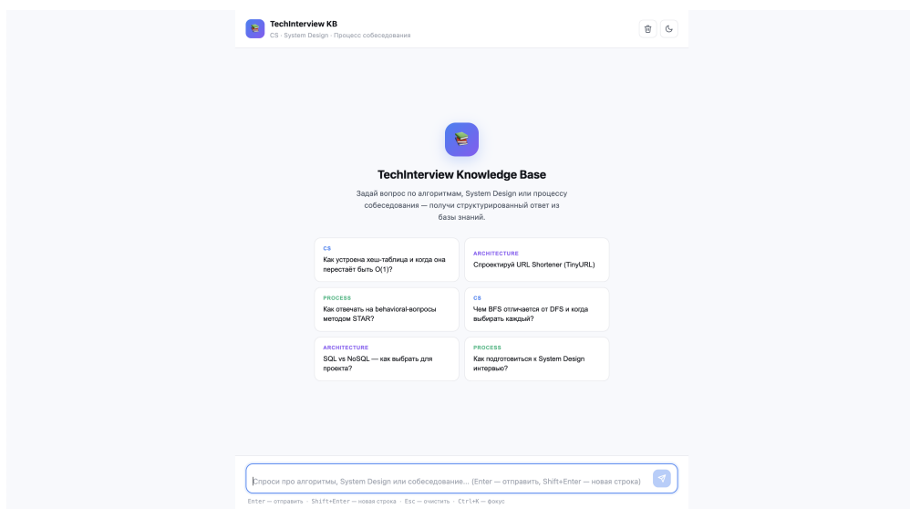
Рисунок 3.2 – Клиентский интерфейс веб-MVP: переключатель темы (светлая/тёмная), блок предложенных вопросов и функция очистки чата
